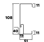
Rysunek techniczny
