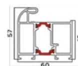
Rysunek techniczny
