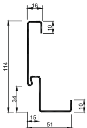
Ościeznica stalowa 11/54, 11/54 ALU
